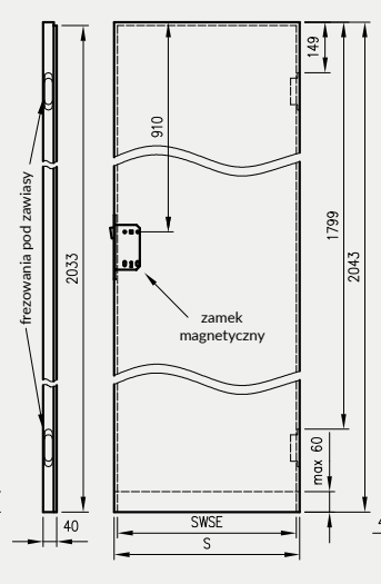
Skrzydła Sara Eco bezprzylgowe
