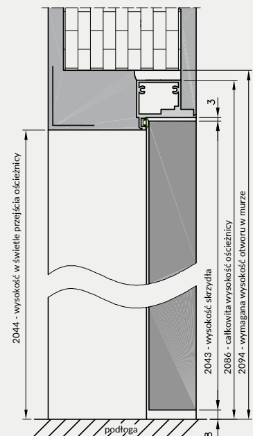
Przekrój pionowy drzwi Sara Eco
