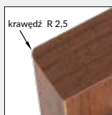
krawędź R 2,5 mm w laminatach CPL
