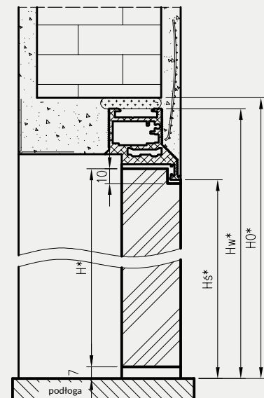
Przekrój pionowy drzwi Sara Eco 2 przylgowe - otwierane do wewnątrz
