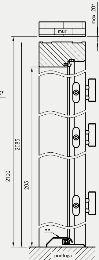
Przekrój pionowy OD ATHOS
