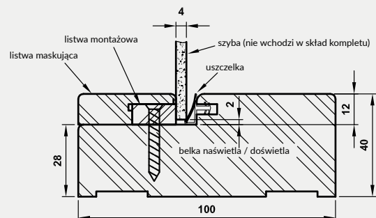
Rys. Przekrój naświetla / doświetla
