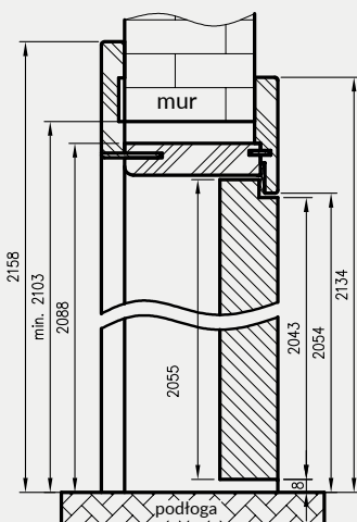
Przekrój pionowy ORO
