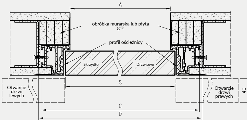
Przekrój poprzeczny drzwi Sara Eco2 bezprzylgowe - otwierane na zewnątrz
