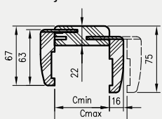
Przekrój TUN z ką. T80
