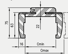
Przekrój OR/ORC Natura z ką. N63
