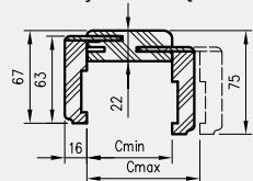
Przekrój TUN Natura z ką. N63
