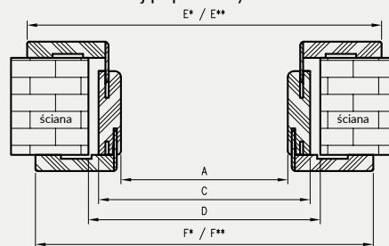
Przekrój poprzeczny TUN
