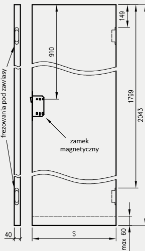
Skrzydła Sara Eco bezprzylgowe
