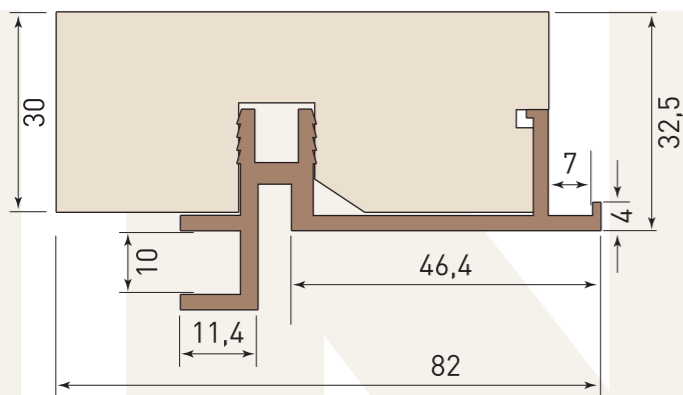
SYSTEM OTWIERANIA INVISIBLE
