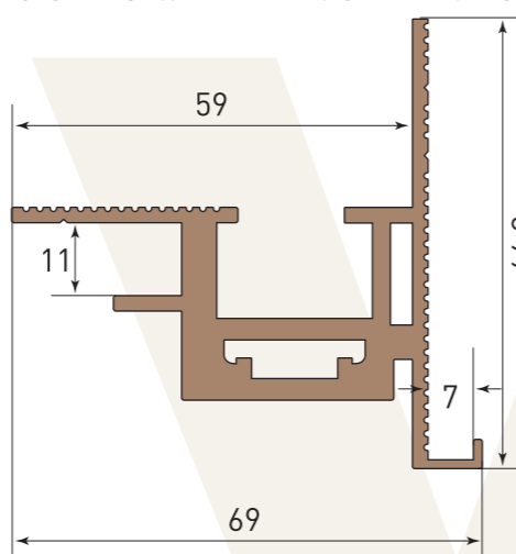
SYSTEM OTWIERANIA INVISIBLE REVERS
